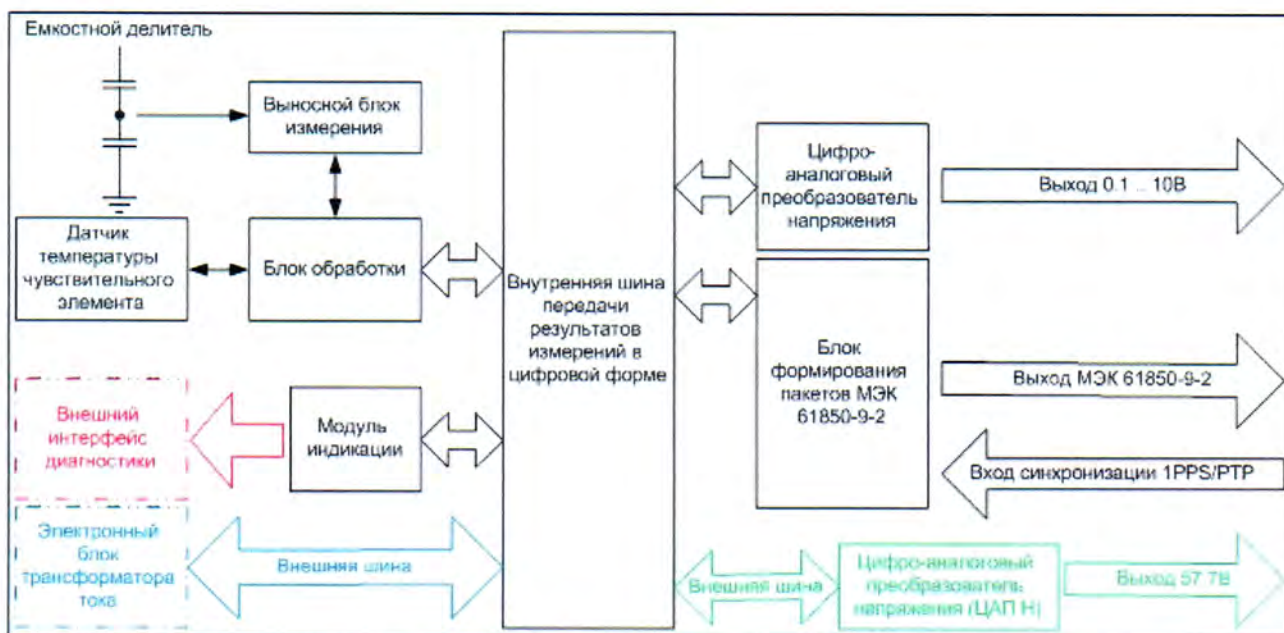
Рисунок 1 - Логическая схема ДНЕЭ
